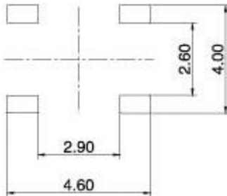
P.C.B diagram
