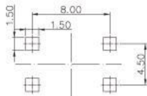
P.C.B焊接图 P.C.B diagram
