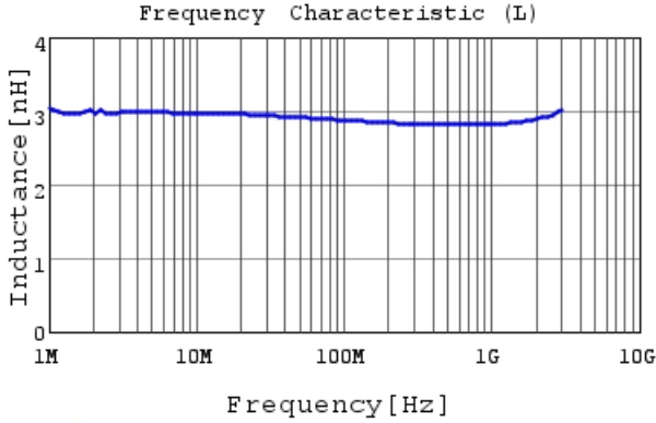
LQW15AN2N9G80 L
