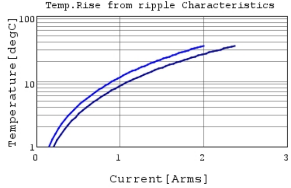
GRM155R70J105MA12 Temp.rise — 500kHz —
