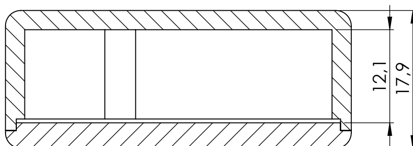
PRZEKRÓJ A-A
