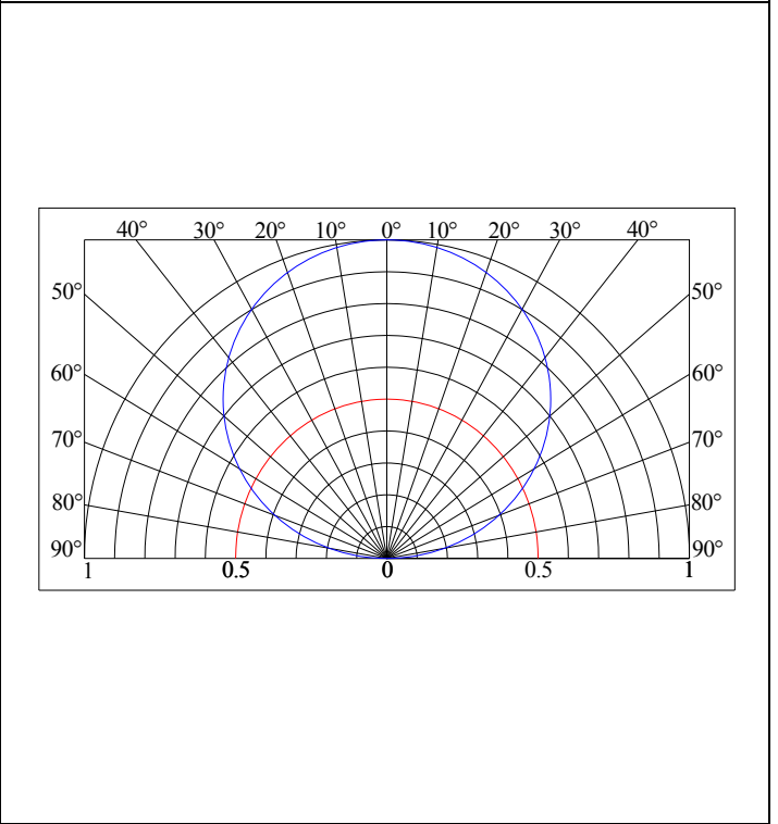
RADIATION DIAGRAM 视角图
