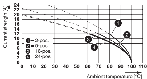
Typ: MSTBP 2,5/...-ST z MSTBA 2,5/...-G-5,08
