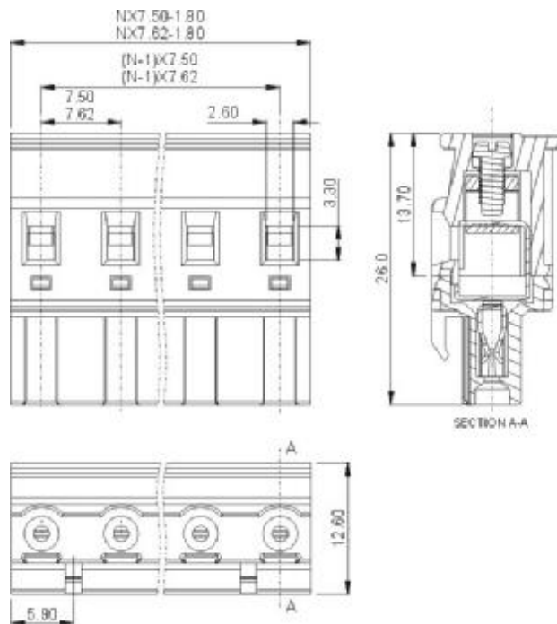
2EDGKB-7.5 2EDGKB-7.62
